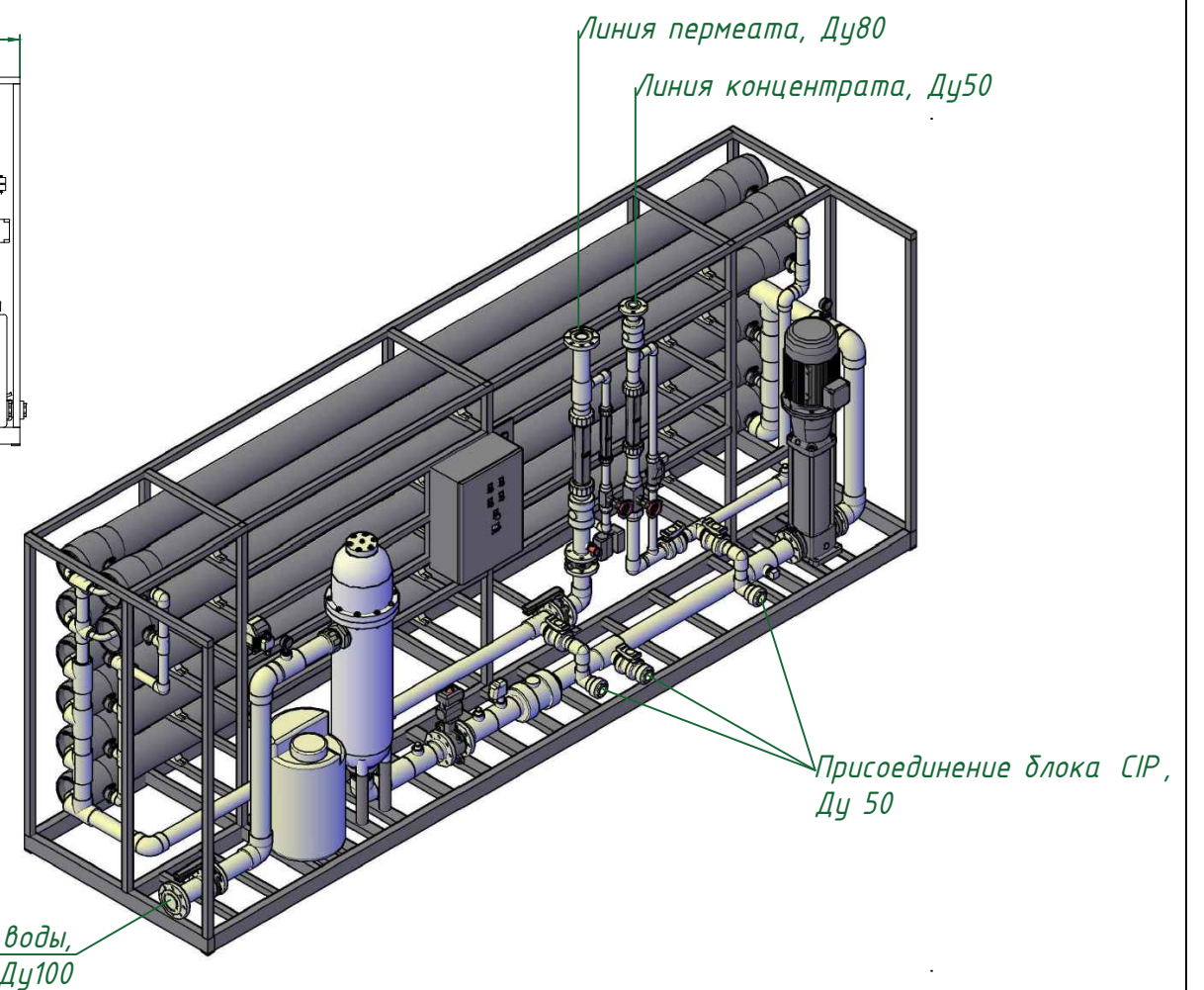
Изометрия
