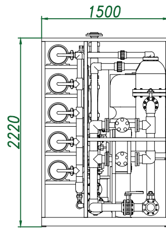
Вид слева
