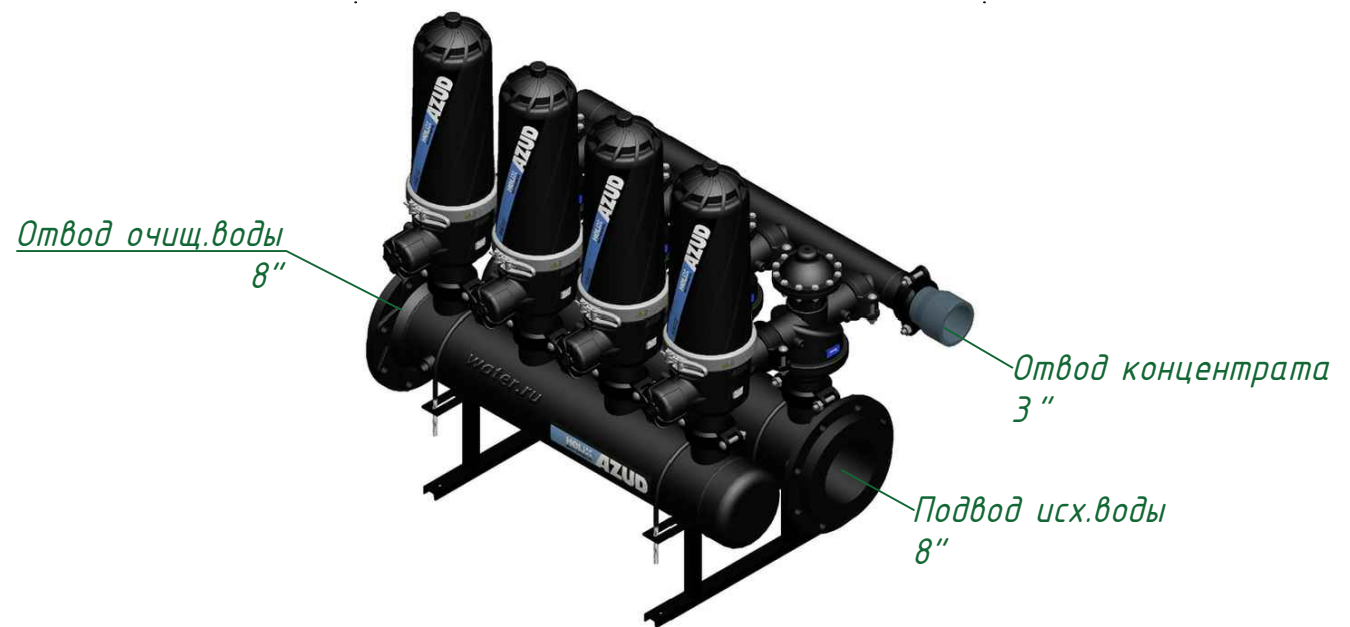
Изометрия
