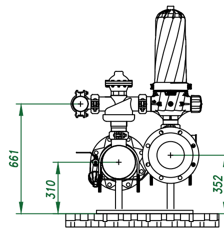
Вид слева
