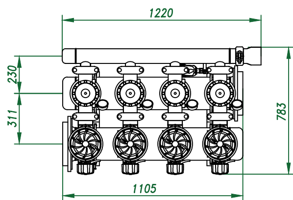
Вид сверху
