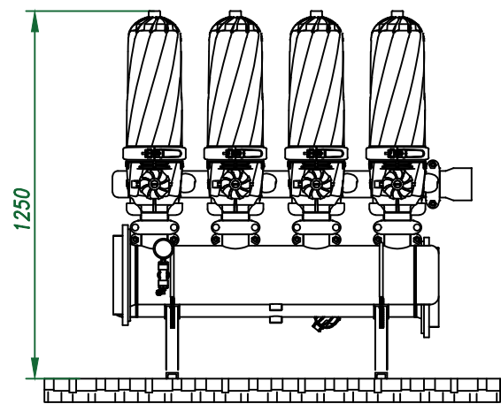
Вид спереди
